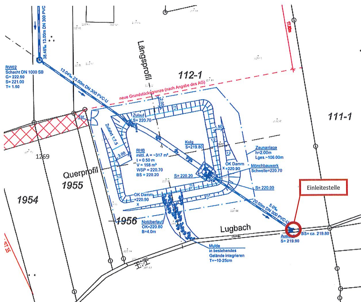
Abbildung 1: Lageplanauszug aus Caigos-Kanaldatenbank
