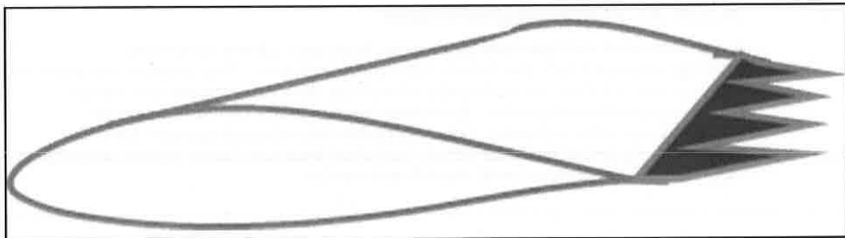
Abb. 2: Prinzipskizze Serrations
