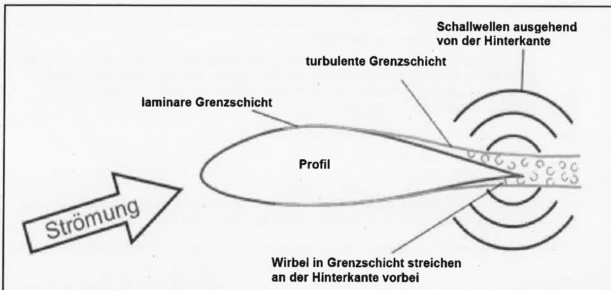
Abb. 1: Skizze zur Entstehung Hinterkantenschall am Rotorblattprofil
