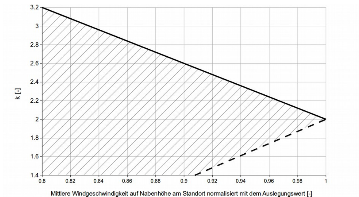
Abbildung 2.1.2: Mögliche Kombinationen von normierter Windgeschwindigkeit und Formparameter k der Weibull-Verteilung (schraffierter Bereich).
